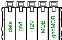
Récepteur radio
